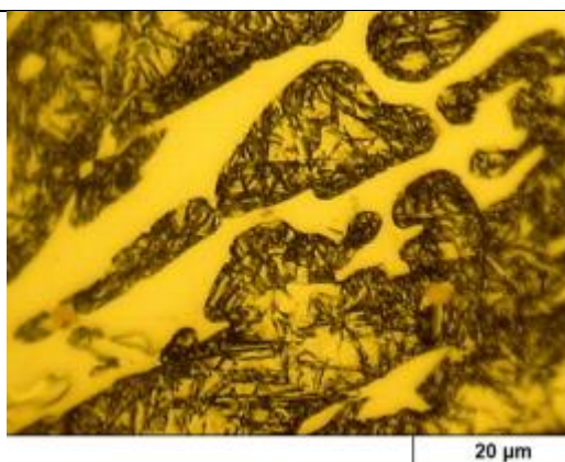
کاربید در زمینه مارتنزیت به همراه مقادیری آستنیت باقیمانده
