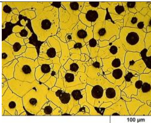
گرافیت های کروی در یک نمونه چدن نشکن با ساختار فریت به همراه نواحی پرلیت
