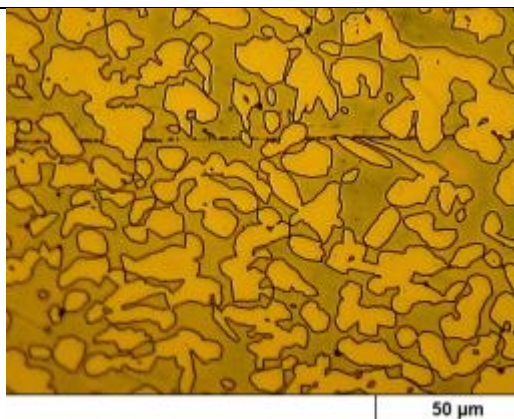
ساختار دایپلکس حاوی فریت و آستنیت
